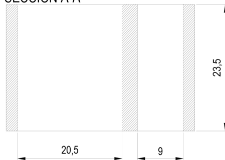
SECCION A-A
